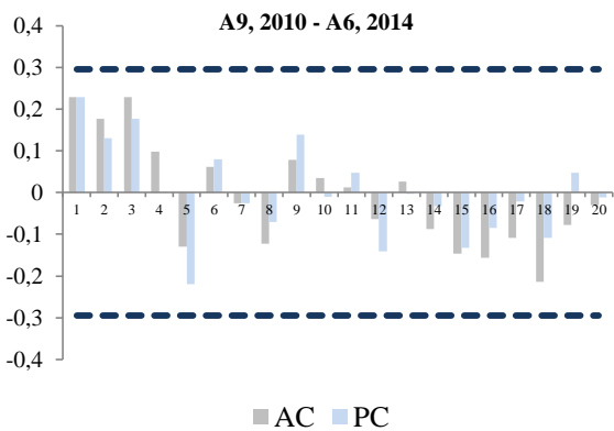
Şəkil 9. Avtokorrelasiya funksiyası (inflasiya)
